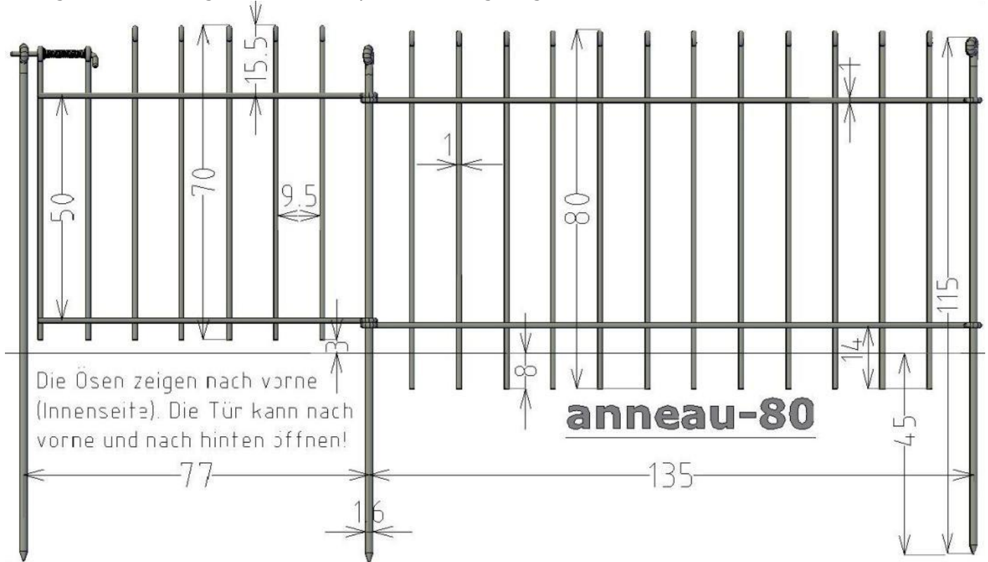
Zeichnung vom Steckzaun Modell anneau-80-... mit Tür (Maße in cm)
